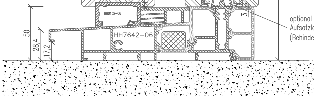
Schnitt A-A
