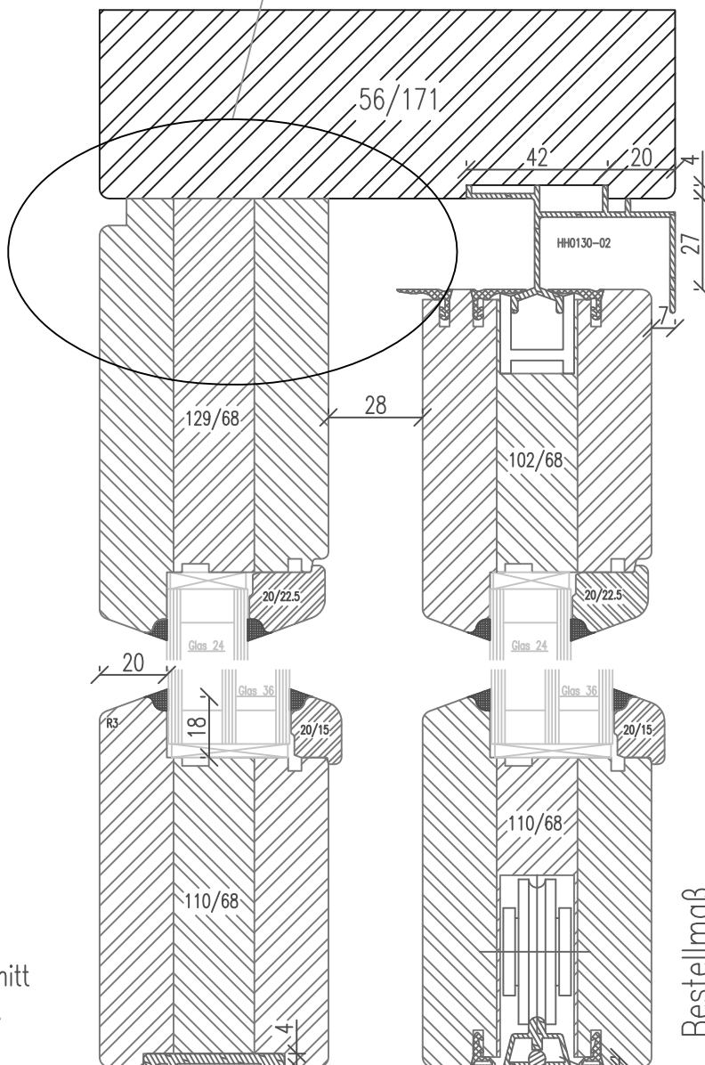
Schnitt C-C
